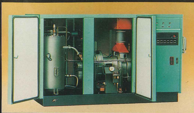
LGII 12A-3/7-D型低噪聲螺桿壓縮機
